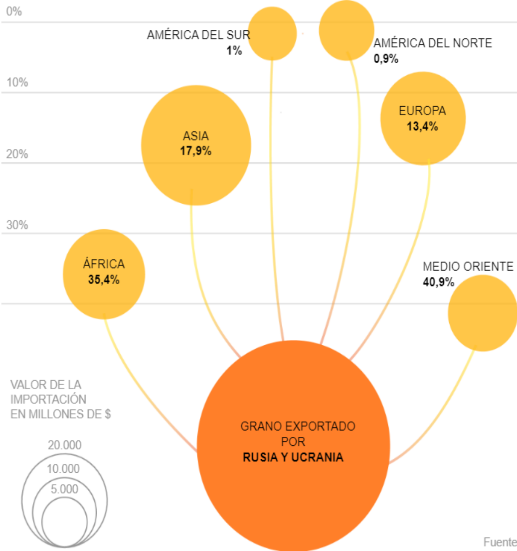
El PESO DEL GRANO DE UCRANIA Y RUSIA EN PORCENTAJE
